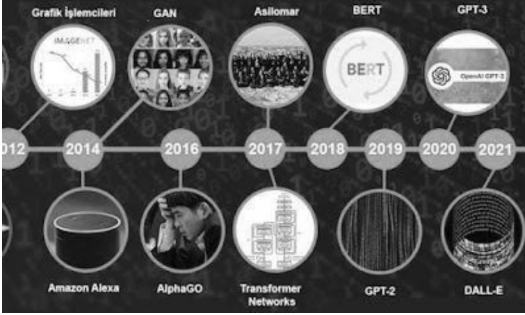
yapay-zekâ-zaman-cizelgesi (2012-2021)
